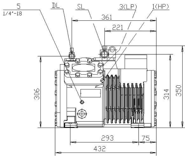
Чертеж компрессора BS-SH-4L3-18E
