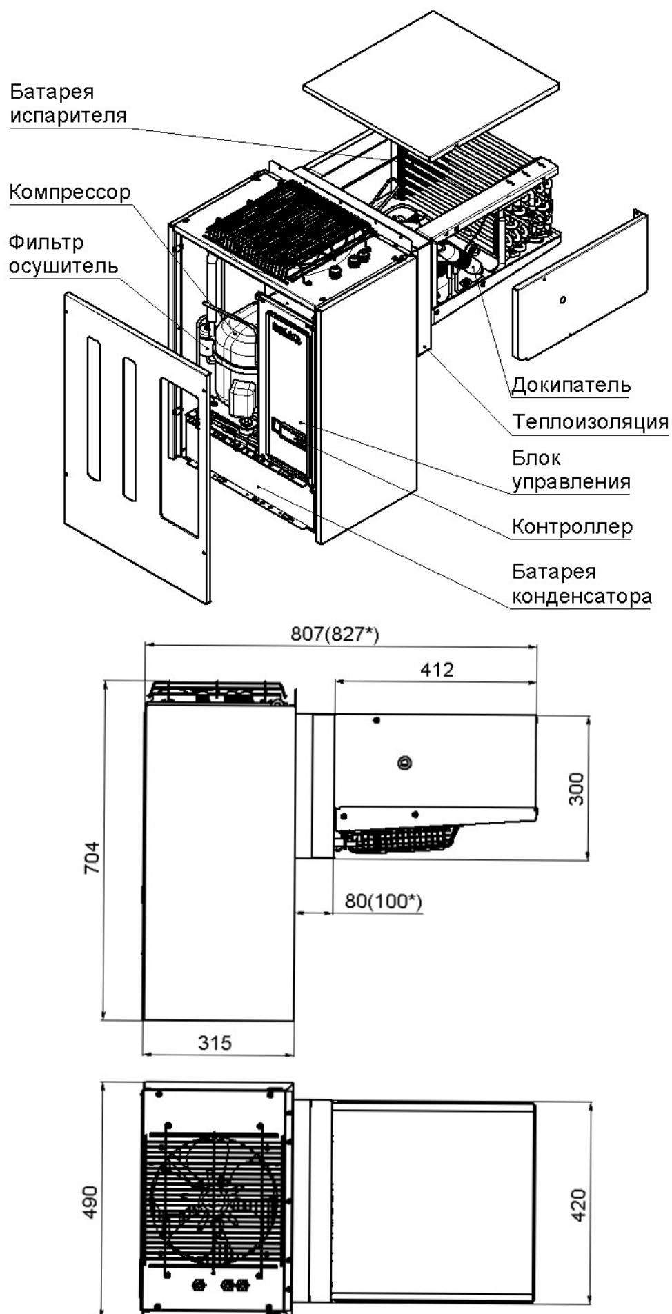
Рис.1 Общий вид и габаритные размеры холодильной машины (моноблока) 121 серии: * - Низкотемпературные холодильные машины
