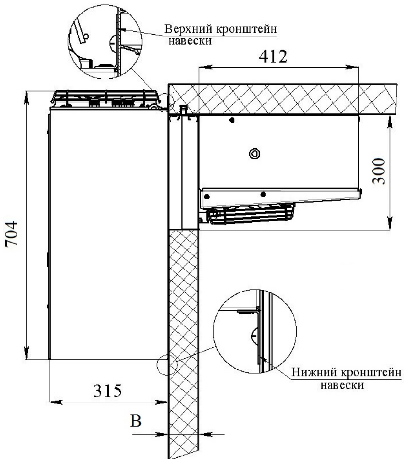
Рис.4 Схема установки моноблока 121 и 221 серии.
