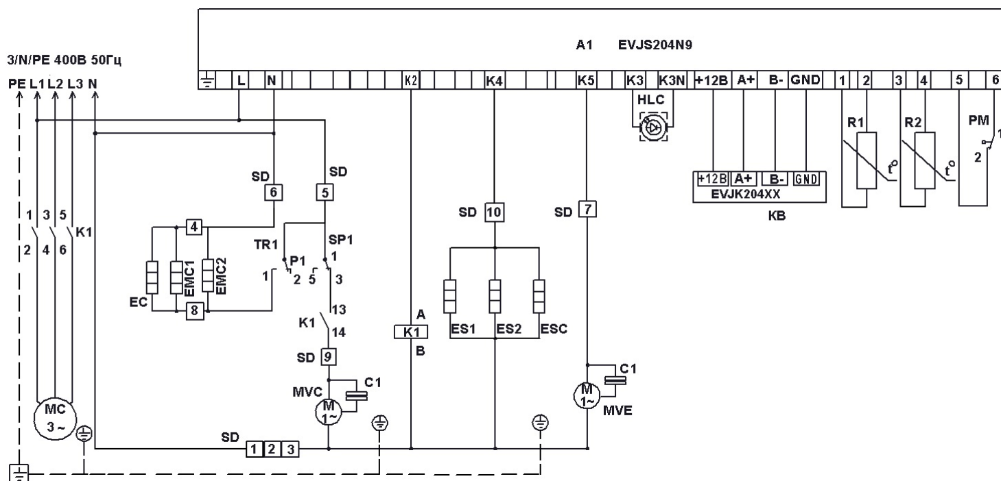
Рис.12 Схема электрическая принципиальная моноблоков MM3...SDU, MB3...SDU
