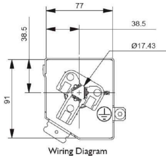
Рисунок 4 Подключение клемм двигателя
