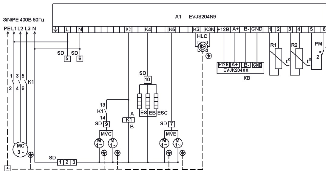
Рис.1. (трехфазное питание)
