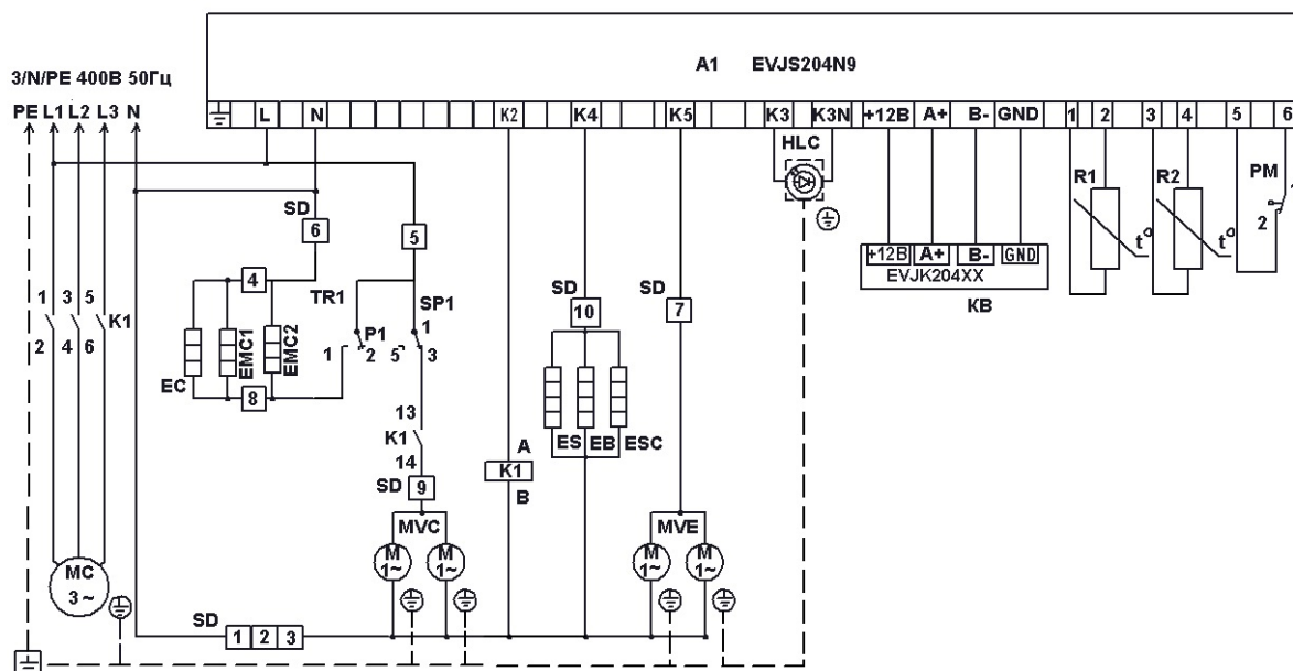
Рис.1. (трехфазное питание)
