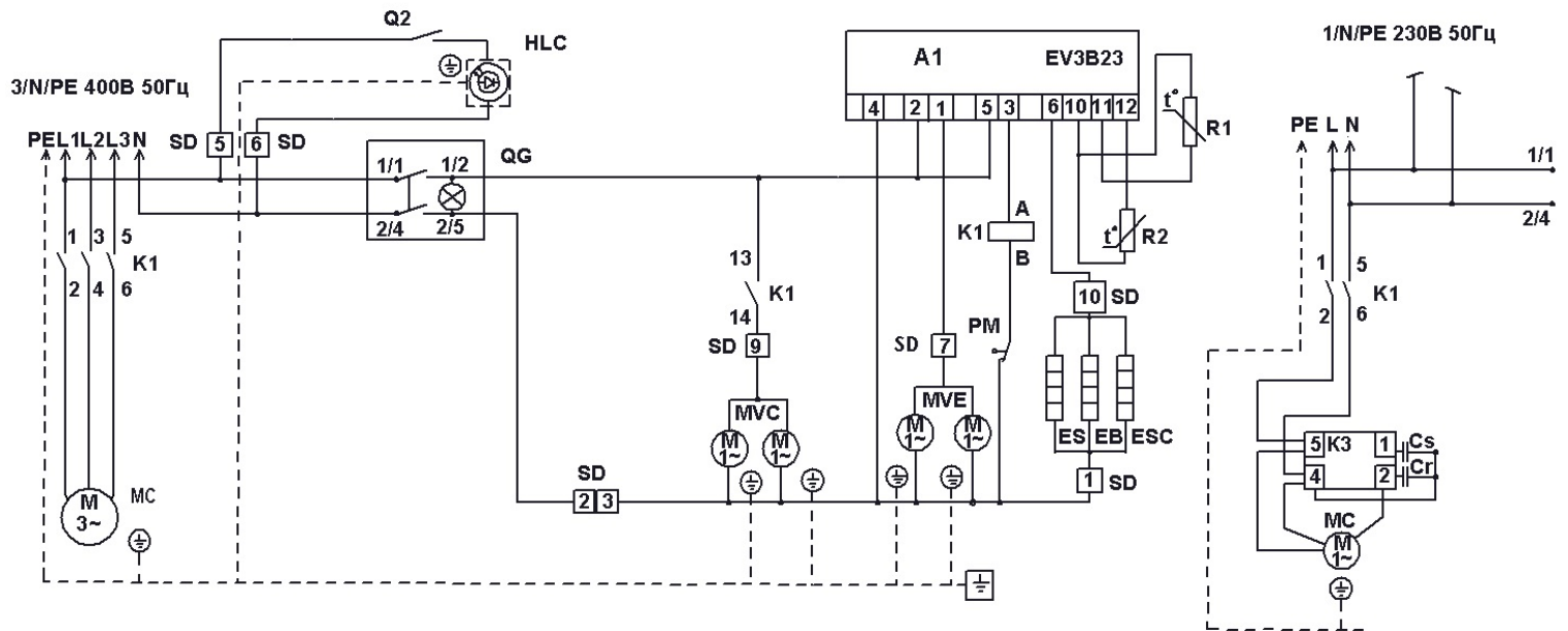
Рис.2 (однофазное питание) остальное см. рис.1
