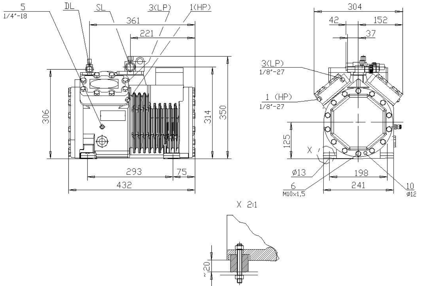
Чертеж компрессора BS-SH-4L4-22E
