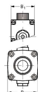
DEV S25 DEV S32 DEV S40结构示意图
