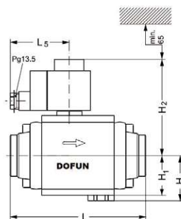
DEV S25 DEV S32 DEV S40结构示意图
